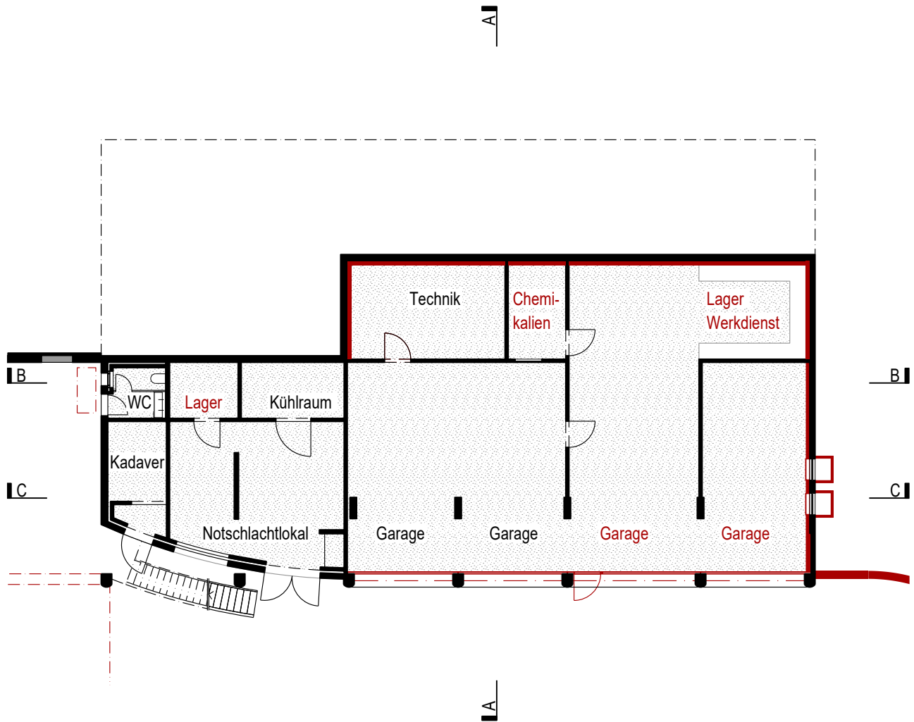
Grundriss Untergeschoss
