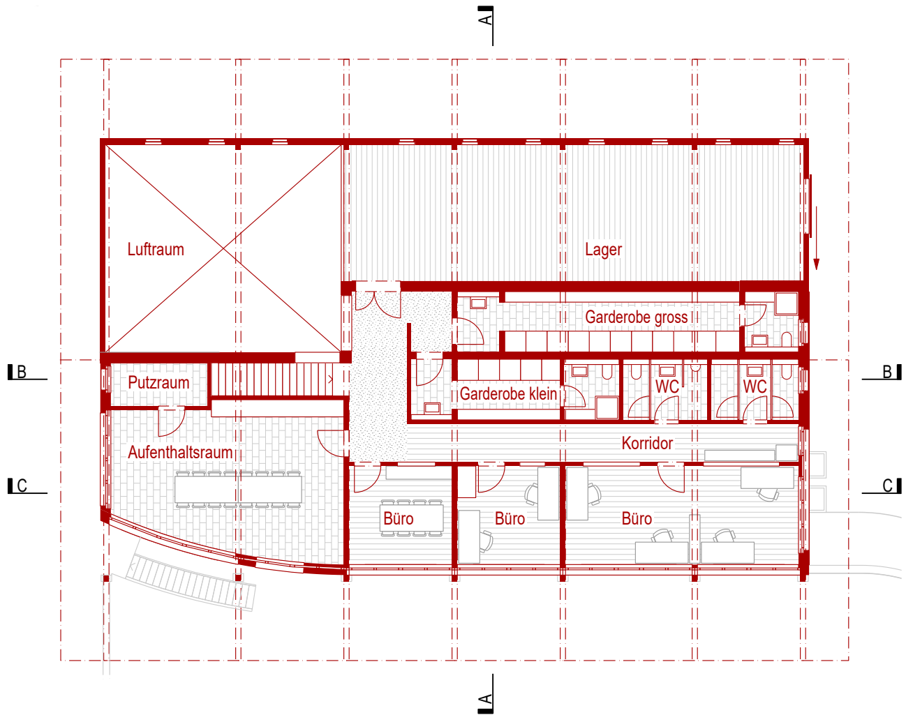
Grundriss Obergeschoss
